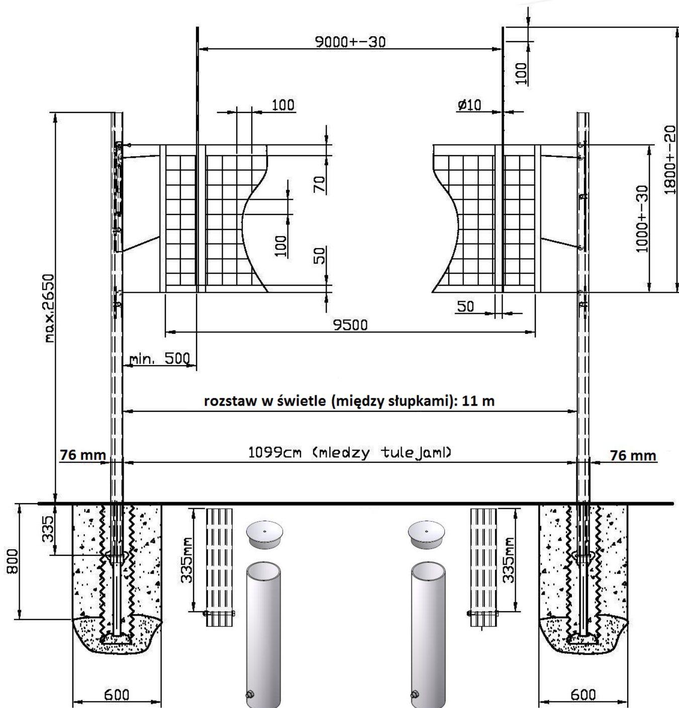
RYSUNEK NR 1 – ZESTAW DO SIATKÓWKI
